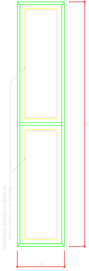
CAIXA DE LUZ ESTRUTURA
